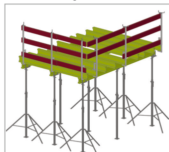
Deckenschalung
